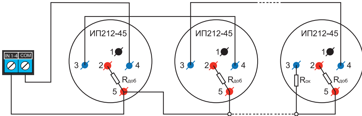
Рисунок 2. Схема подключения ИП212-45 к пожарному входу NV 2104 с добавочными и с оконечным резисторами
