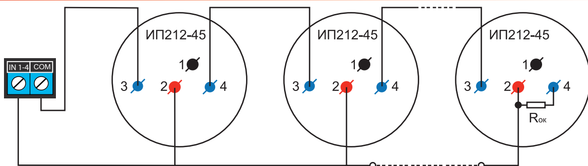
Рисунок 3. Схема подключения ИП212-45 к пожарному входу NV 2104 только с оконечным резистором
