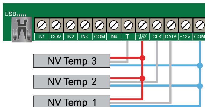
Рисунок 2. Подключение датчиков температуры NV TEMP
